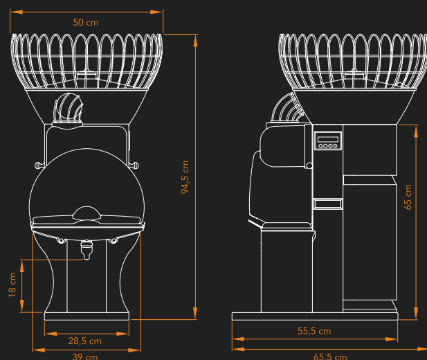
CITROCASA Fantastic F/SB ADVANCE – Technische Spezifikationen
