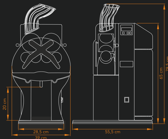
CITROCASA Fantastic M/AS ADVANCE – Technische Spezifikationen
