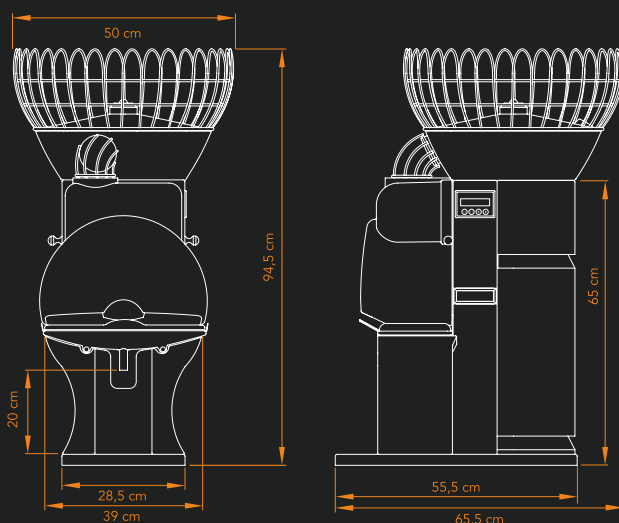
CITROCASA Fantastic F/D ADVANCE – Technische Spezifikationen
