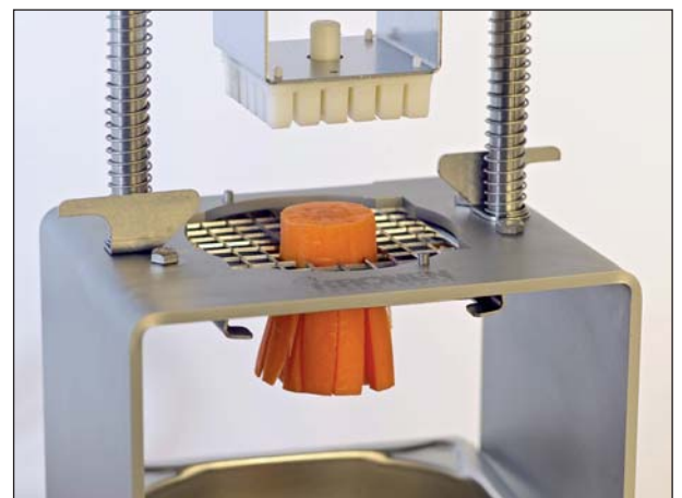
Stickstecher für Karotten und Kohlrabi 10 x 10 mm
